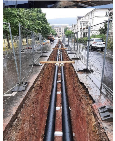
Hauptleitung DN200, Charlottenstraße Foto: Stadtwerke Meiningen GmbH
